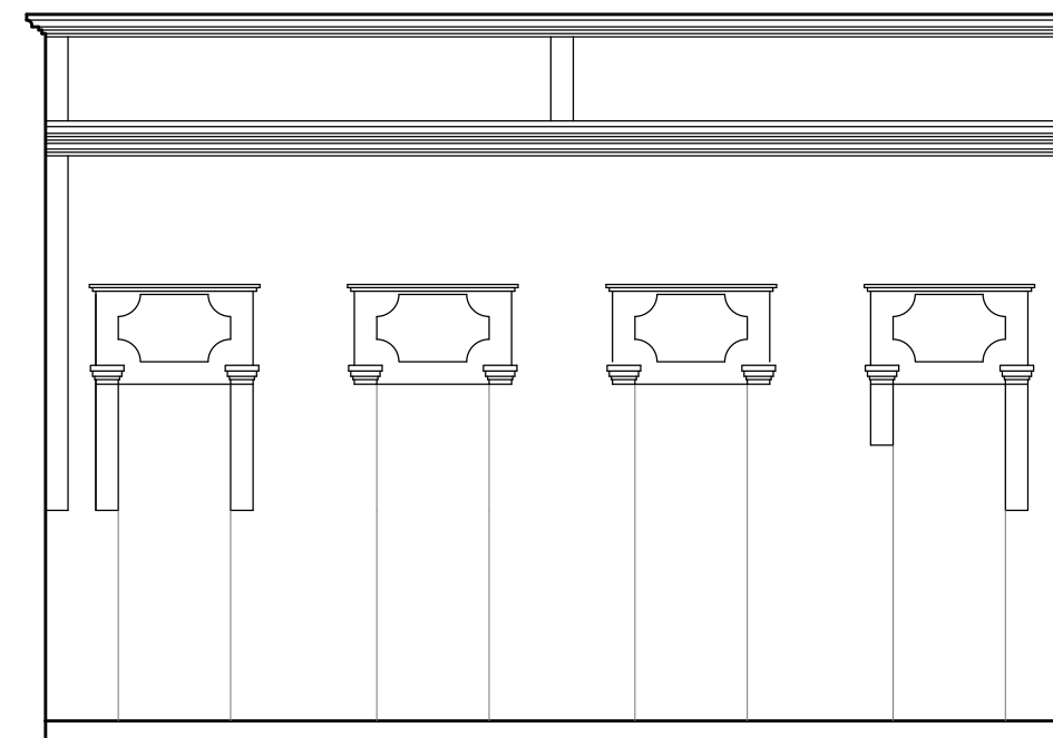
EDIFICAÇÃO RC-251 FACHADA FRONTAL ESC. 1/75
