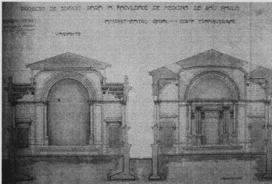
Corte do Teatro – estudo da Comissão de Obras da Faculdade de Medicina Arquivo Museu Histórico FMUSP
