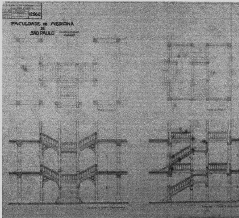
Desenhos originais da escada central do edifício Arquivo Condephaat
