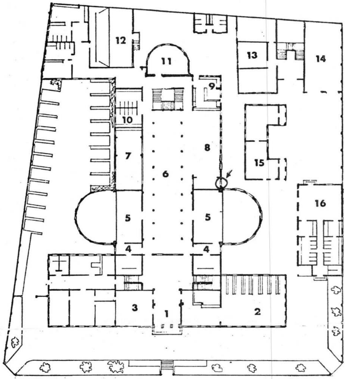
PLANTA D TÉRREO ESC.1:50C
