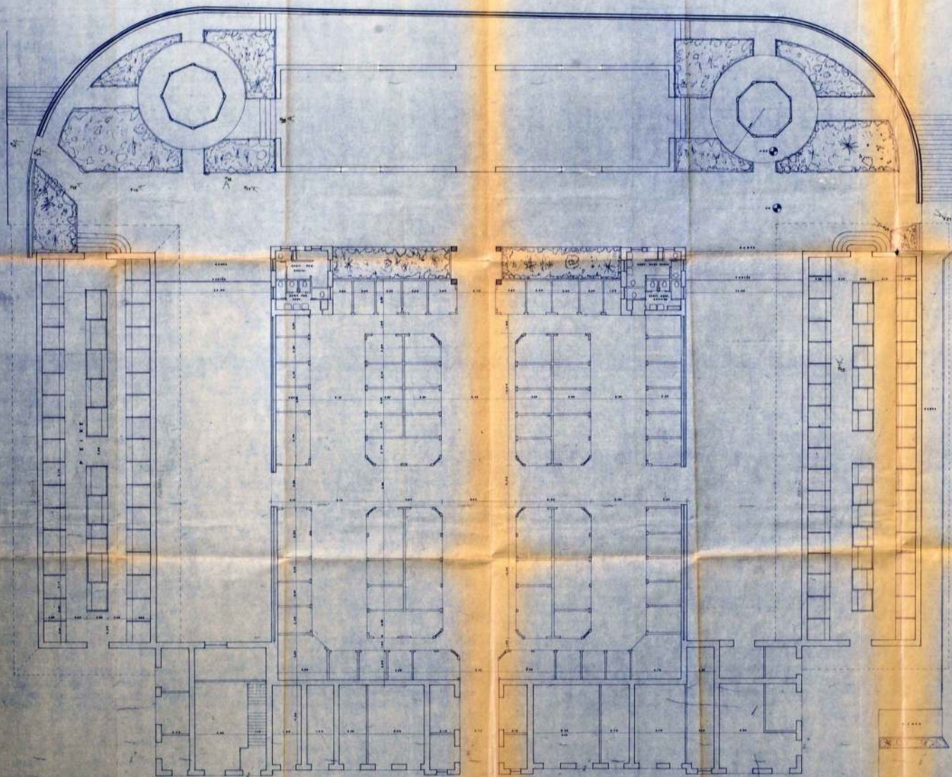
PLANTA BAIXA — MERCADO ADOLPHO LISBOA
