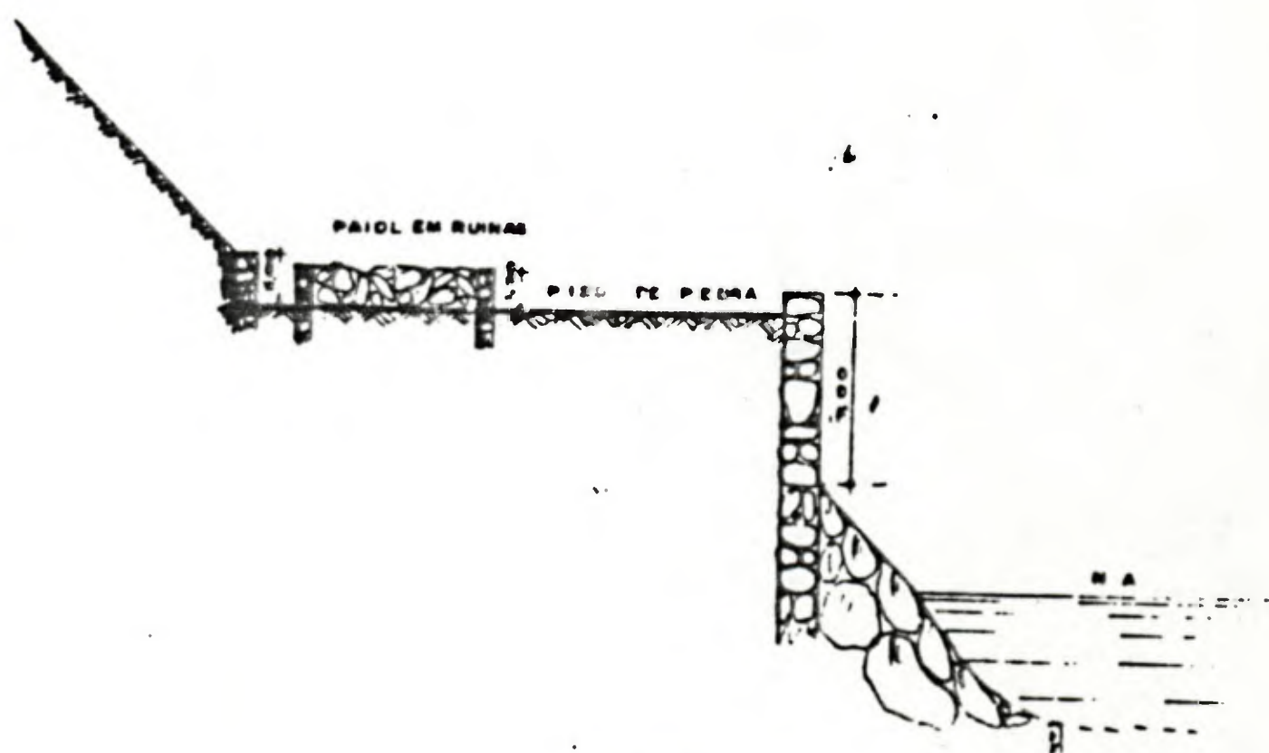
CORTE esc. aprox. 1:500
